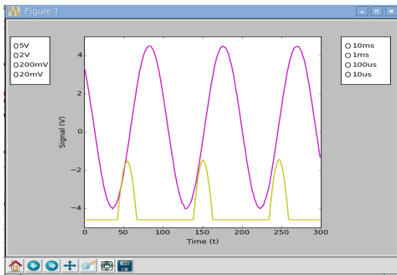
Fig. 5. Sine wave 8Vp-p
